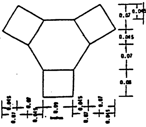
S24 VORTAC SYMBOL
